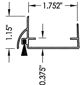
45 DOOR SWEEP
